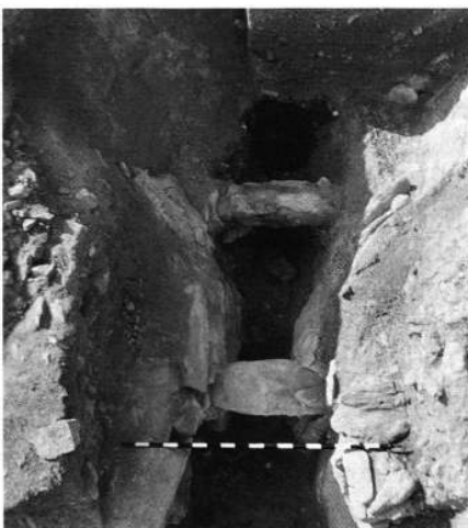
9: Sicht auf Ofen 3 (südwestlicher Viertel noch nicht ausgegraben). In der Mitte des kanalartigen Feuerraumes das aus Pfeilern und Steinsturz bestehende Auflager des Rostes. Vue générale du four 3. Le quart sud-ouest du four n'a pas été dégagé. Les éléments de soutènement de la sole (deux bases espacées) sont visibles au centre de la chambre de chauffe en forme de couloir. Vue verticale.
